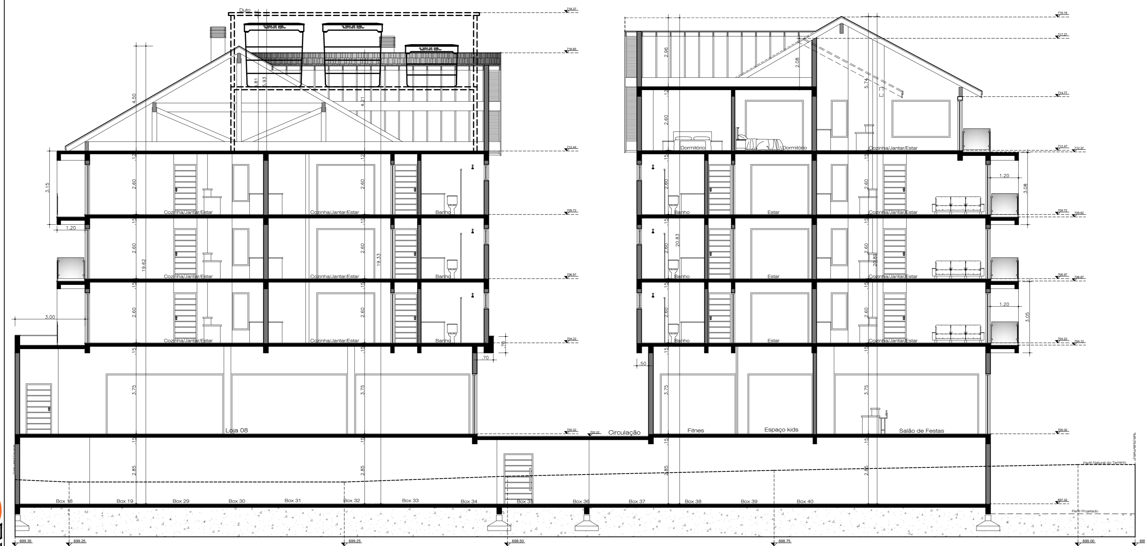
Corte B-B
