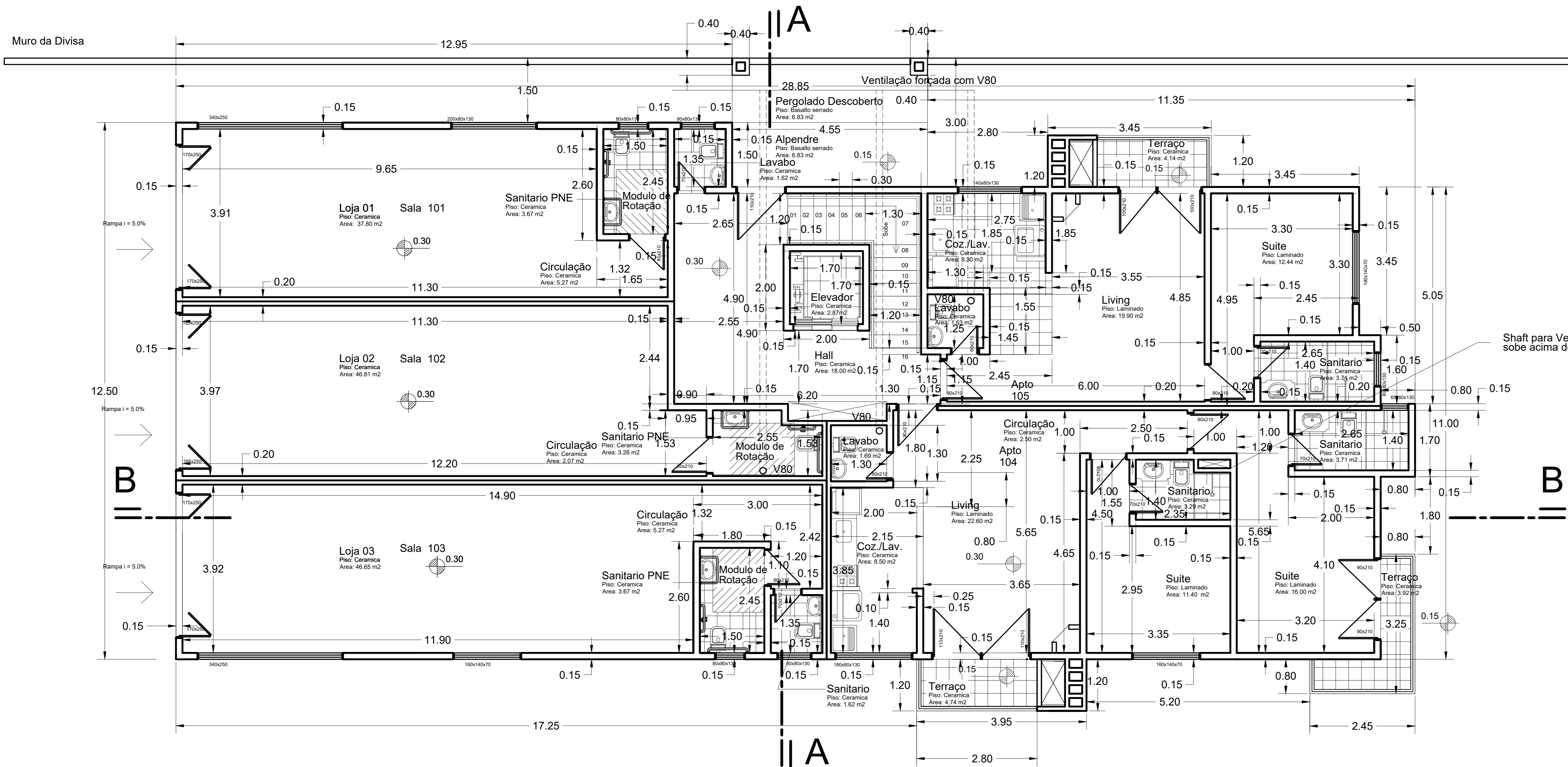
PLANTA BAIXA TERREO Área.: 347.50 m 2 Esc.: 1/50
