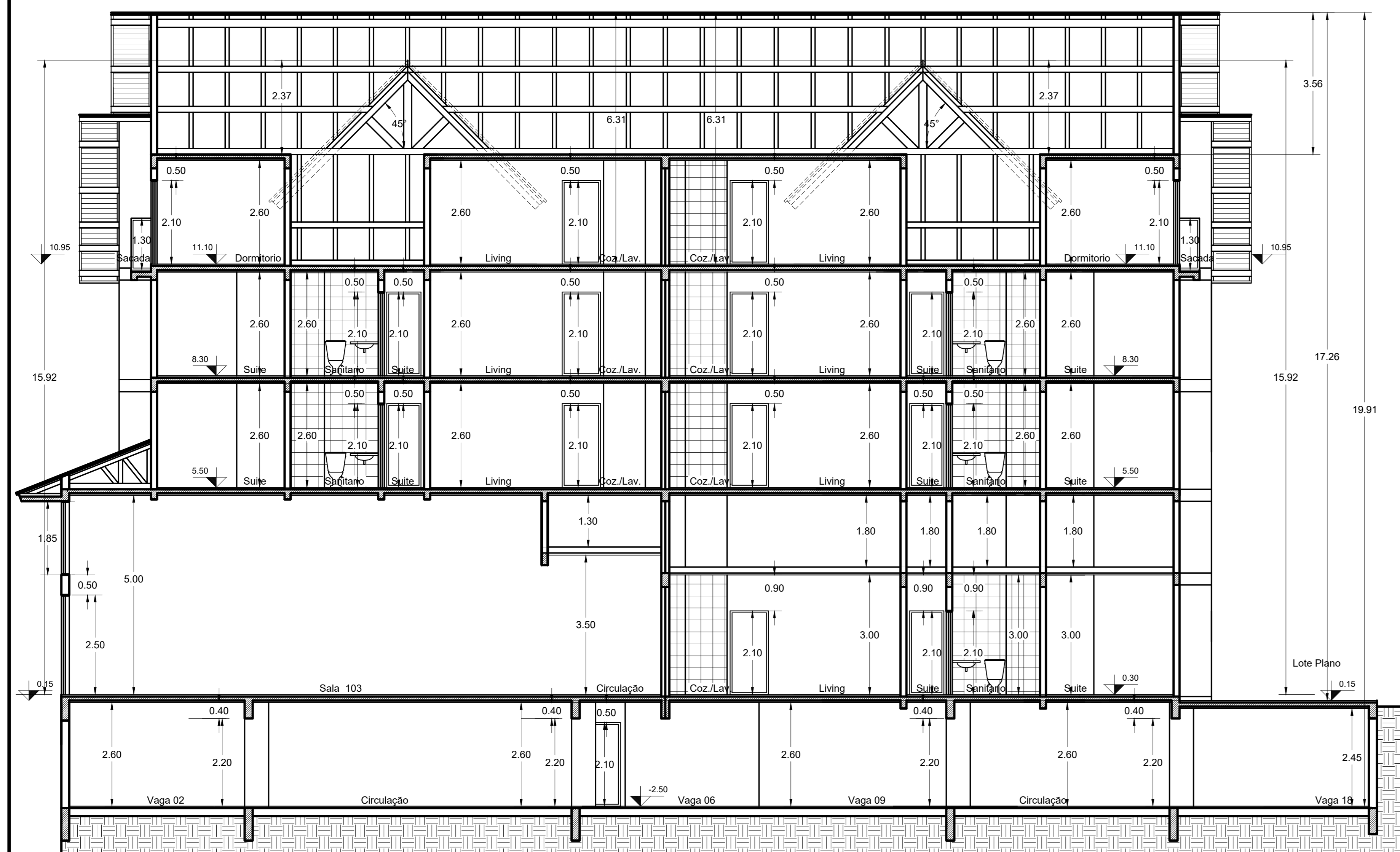
CORTE BB
