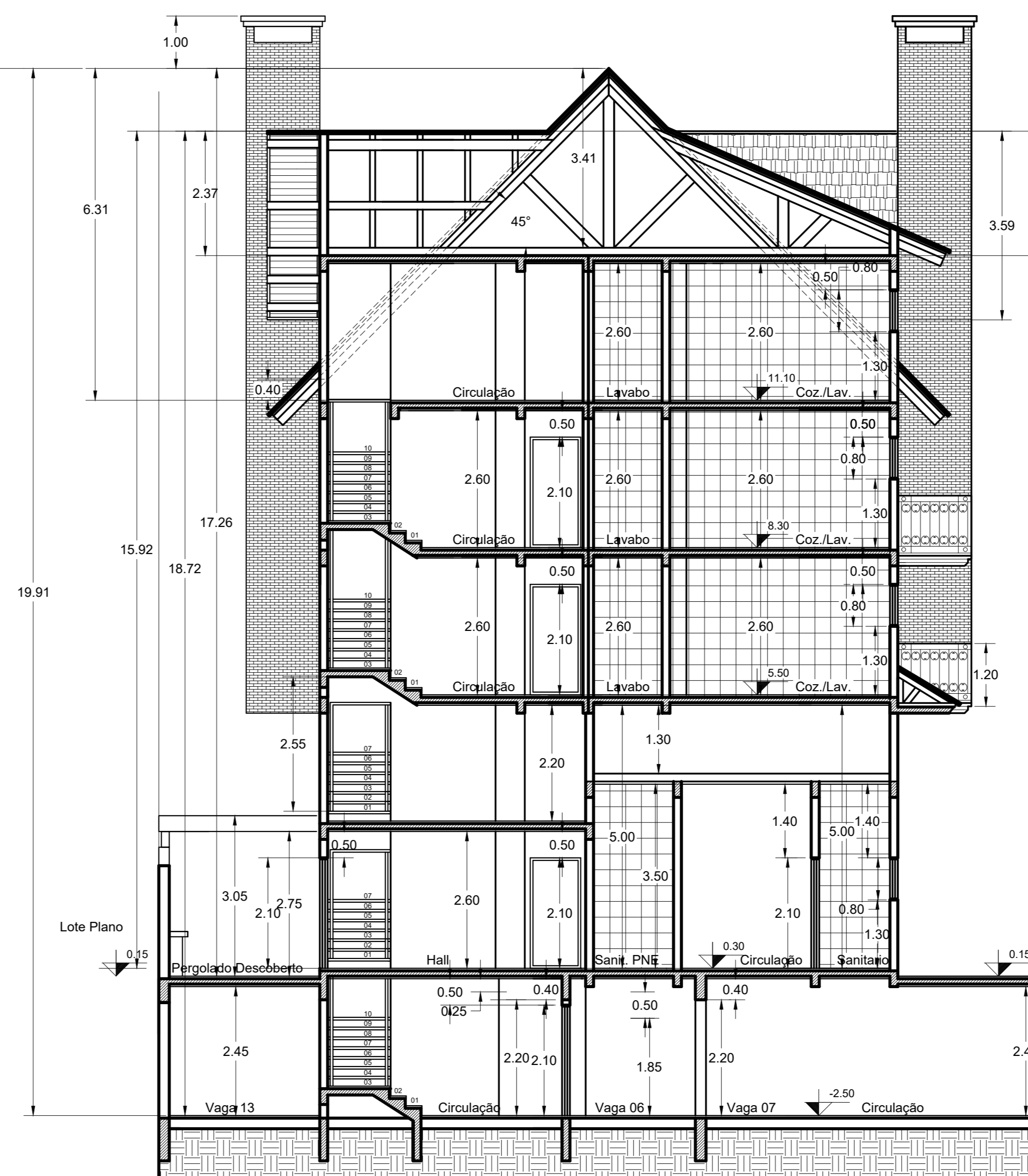
CORTE AA
